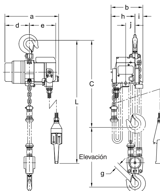
TCR2000P2 Modelo de doble ramal con control de botonera
